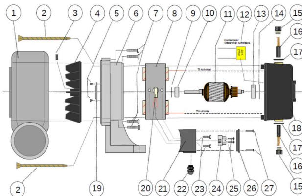
Samletegning til MK 125 - Smedeblæser
